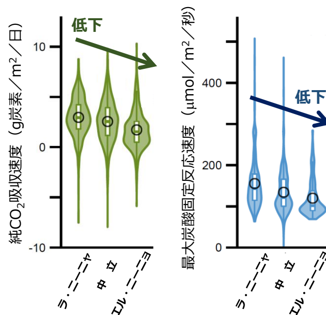
図 3：ボルネオ熱帯雨林のラ・ニーニャ、中立、エル・ニーニョ条件下での森林生産力(純 \text{CO}_2 吸収速度)と Rubisco の最大能力(最大炭酸固定反応速度)
