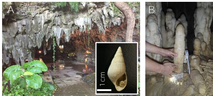
図 1. 沖縄本島南部のサキタリ洞遺跡と出土したカワニナ化石 (A)。同島南部の玉泉洞内で採取された石筍 (B)。
