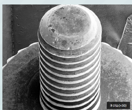
ネジ山 (30倍)
